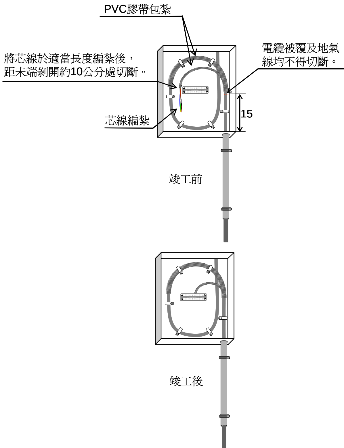
圖(二) 主配線箱施工示意圖
