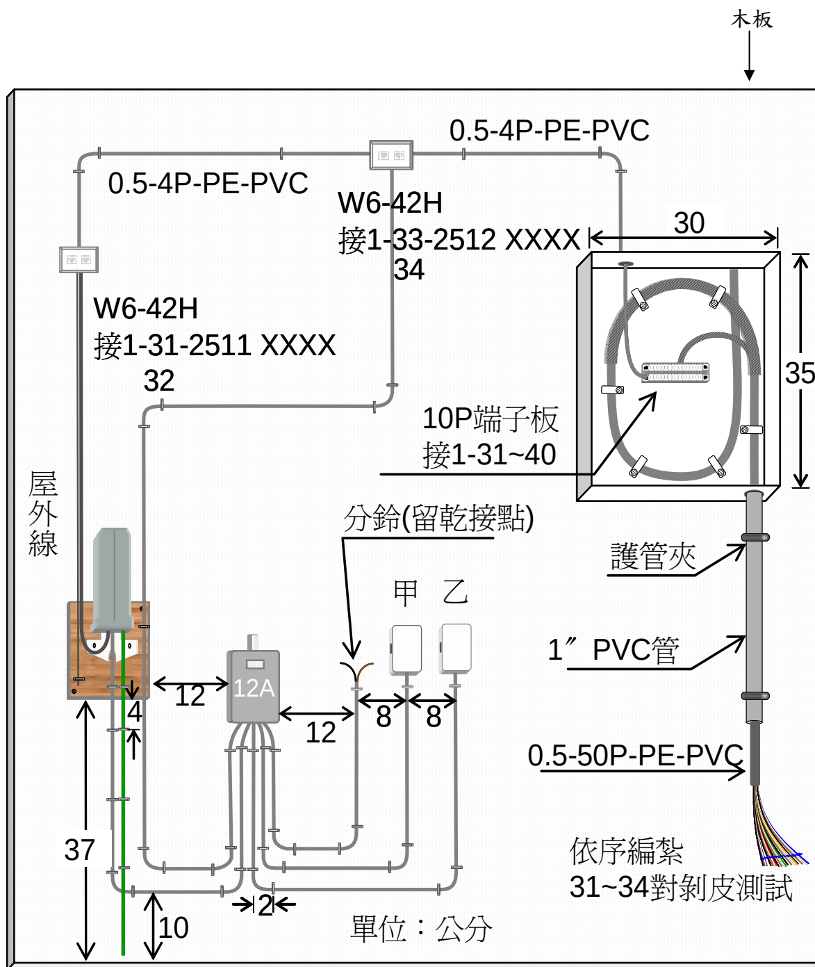
圖(一)主配線箱、配線、及用戶設備裝設示意圖
