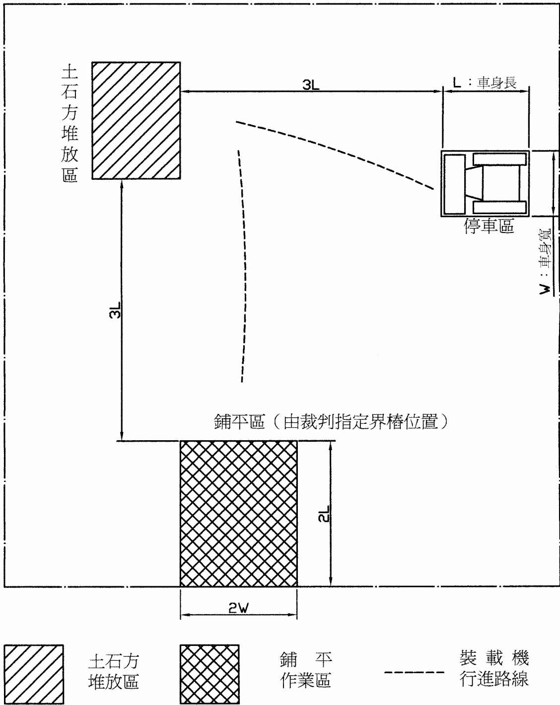
(三) 裝載機鏟料鋪平作業路線圖：07003-930405
