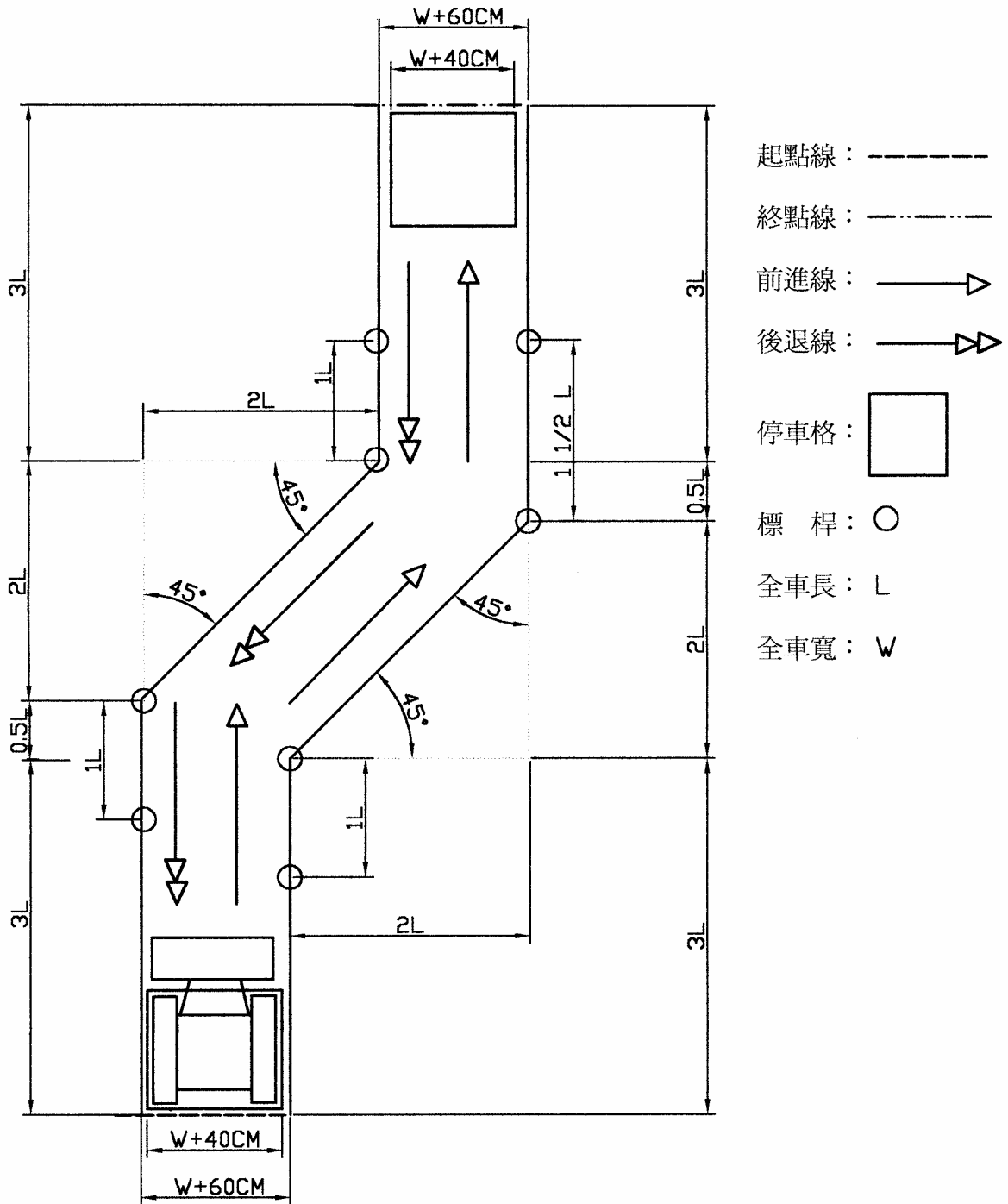
(二) 裝載機樁考場地佈置圖：(07003-930403)
