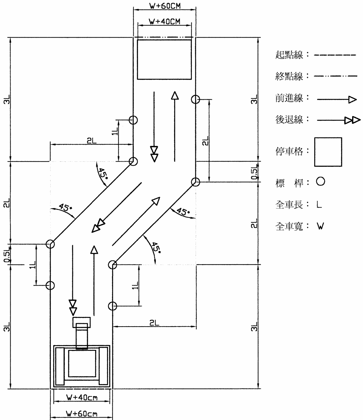
(二) 挖掘機考場地佈置圖：(07002-930403)
