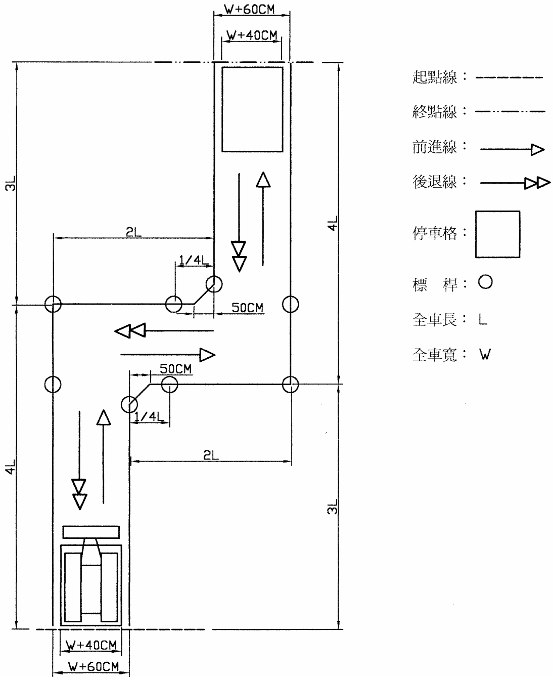
(二) 推土機樁考場地佈置圖：(07001-930403)
