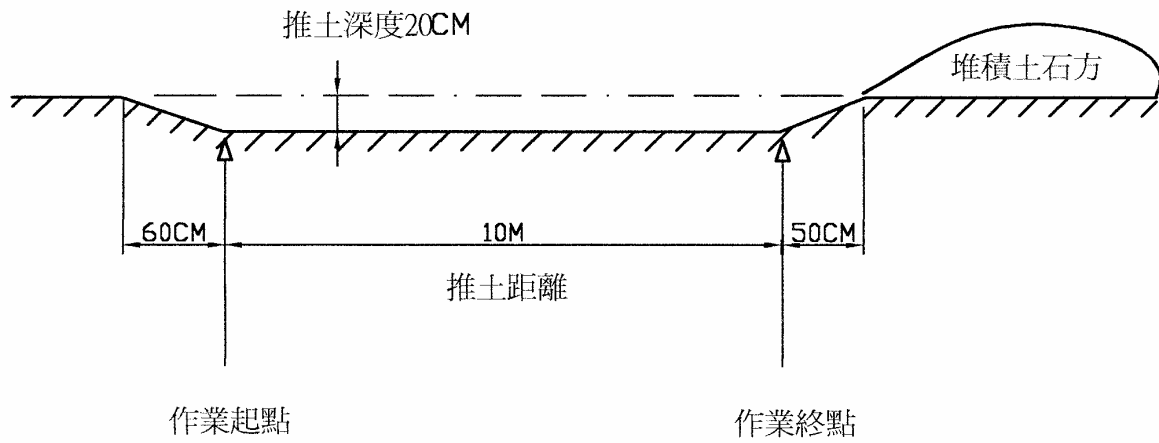
(二) 推土機實地推土作業場地佈置圖(07001-930404)
