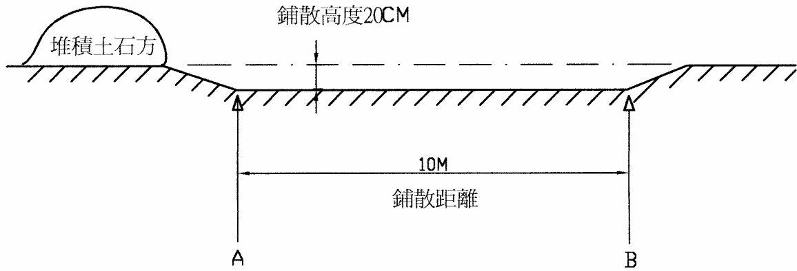
(二) 推土機鋪土推平作業場地佈置圖(07001-930405)
